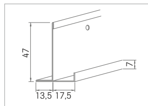
Nr. 8030/15 15er Platte 0,6 mm dick
