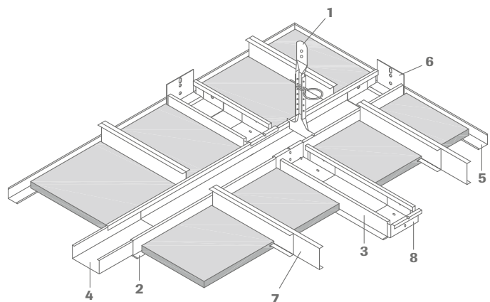
Konstruktionsteile/m 2 (Stückangaben zur passenden Länge)
