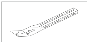
Nr. 17/80 Unterteil für Dreieckaussteifungen
