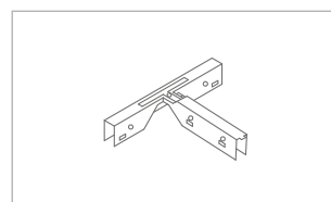
Nr. 61/2 T-Verbinder
