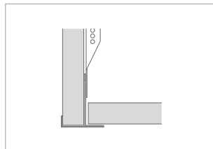
Nr. 8030/13, Nr. 8030/15 Deckenversprung oder Abschottung
