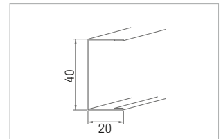
Nr. 57 0,5 mm dick
