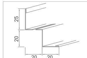
Nr. 56/35 0,6 mm dick (mit Lüftungsschlitzen)
