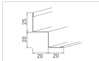
Nr. 56/20 0,6 mm dick Nr. 56/21 1,0 mm dick Nr. 56/23 1,5 mm dick
