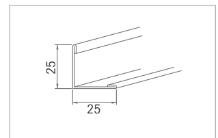
Nr. 51/25 1,0 mm dick
