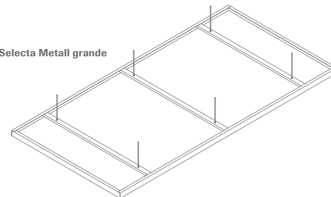
6 Gewindestäbe M6
